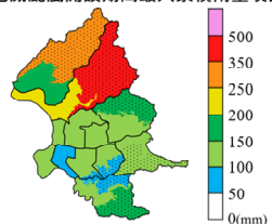
巴威颱風開設期間最大累積雨量填圖
