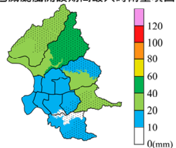
巴威颱風開設期間最大累積雨量填圖
